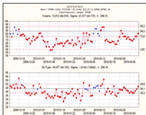
Diagram průměru a směrodatné odchylky jedné z charakteristik elektrolýzy hliníku
